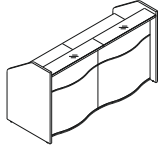
LUV13 1556/770/1103 LUV14 1996/770/1103
