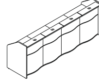
LUV19 3496/770/1103 LUV20 3936/770/1103
